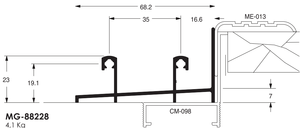
Marco inferior / correr 2
