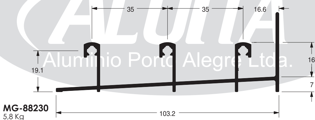
Trilho porta
