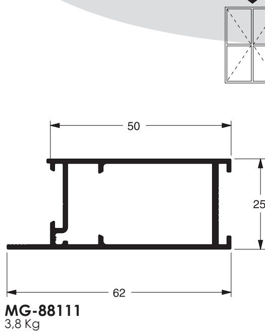
Montante folha
