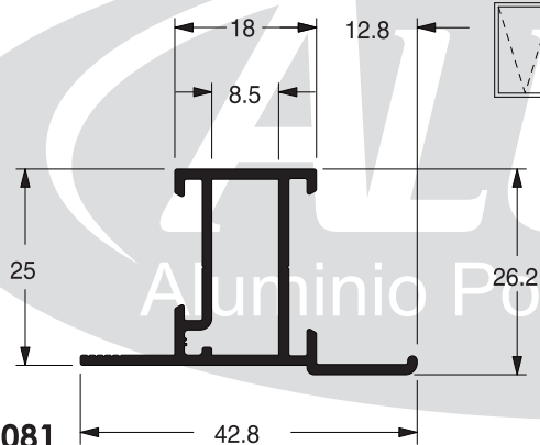
Montante / folha
