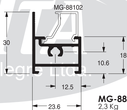
Travessa / folha
