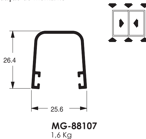
Vedação do montante
