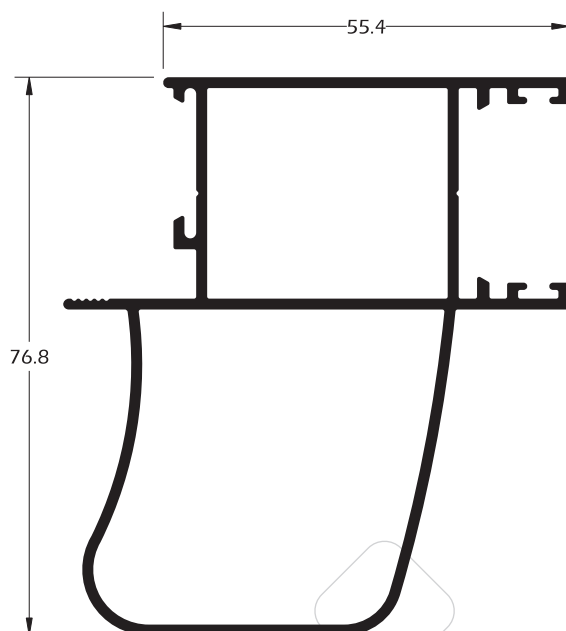
MG-32095 7,9 Kg (5m)
