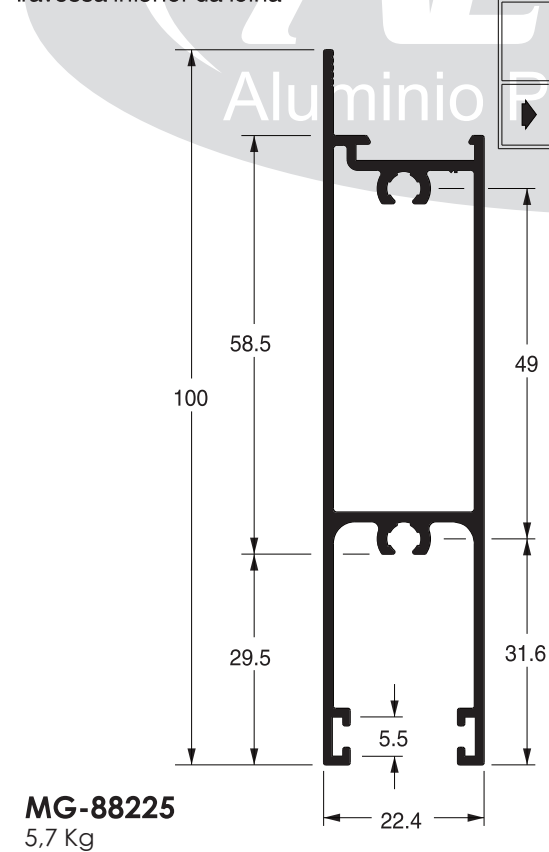
Travessa inferior da folha
