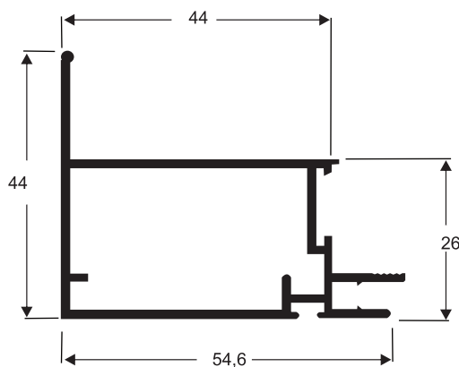
MP-069 3,3 Kg (4,6m)
