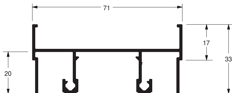
Marco superior / correr 2
