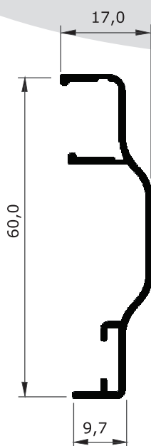
RM-039 (39-1175 C) 1,8 Kg
